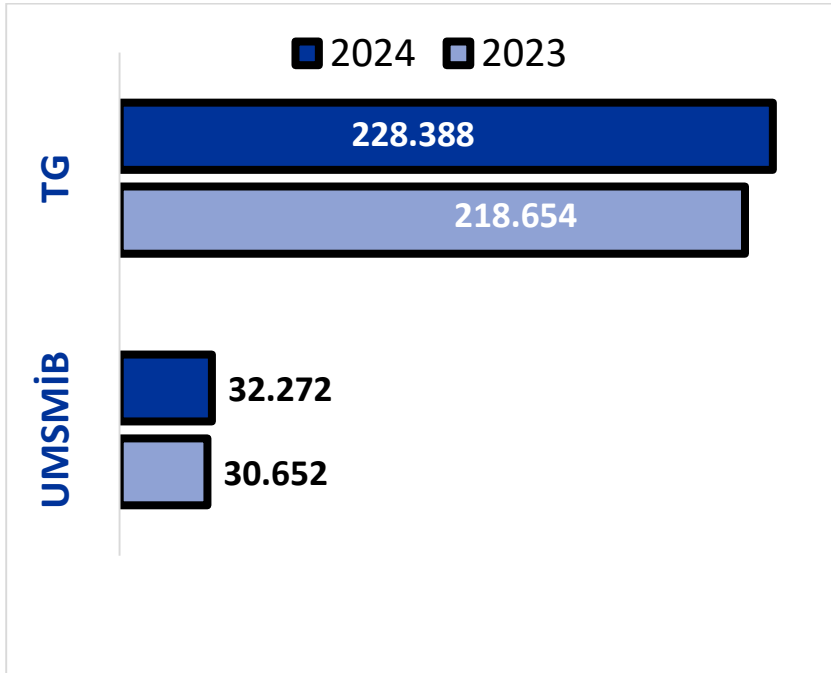
Grafik 1. UMSMİB ve Türkiye Geneli MSM/ Eylül 2024 İhracatı (1.000 $)
